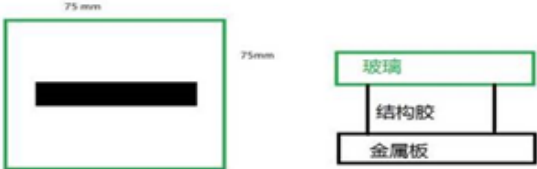
1. 水平方向粘接强度样品示意图
