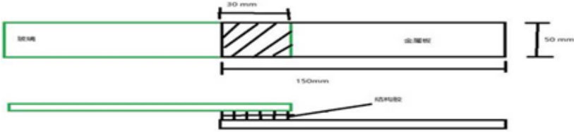
1. 水平方向粘接强度样品示意图
